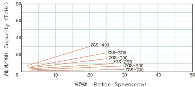
性能参考曲线 Performance diagram
